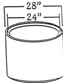
-Manhole Riser w/ Holes~
